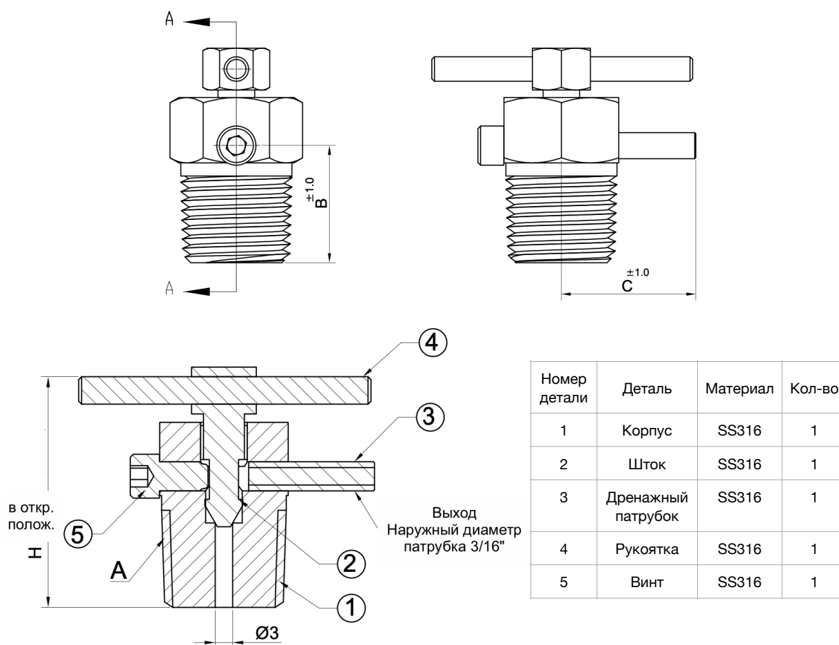
Рисунок 1. Сбросной клапан HAVI BVS-4M-S6-N
