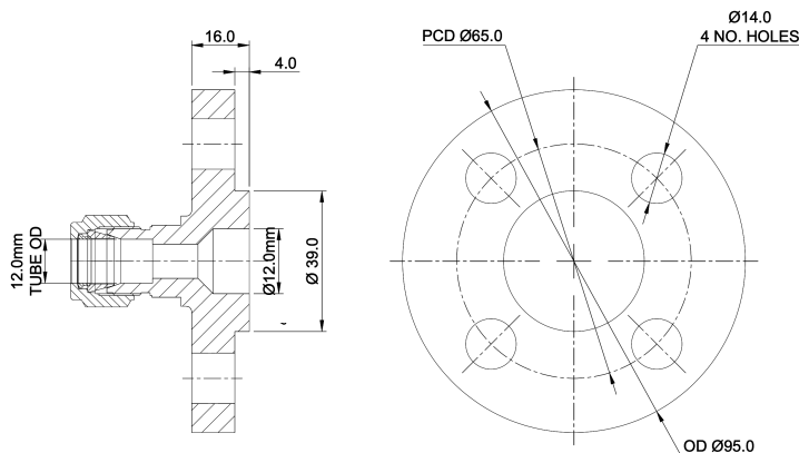
Рисунок 1. Фланцевый соединитель 12MFLADN15PN40-GOSTE-S6
