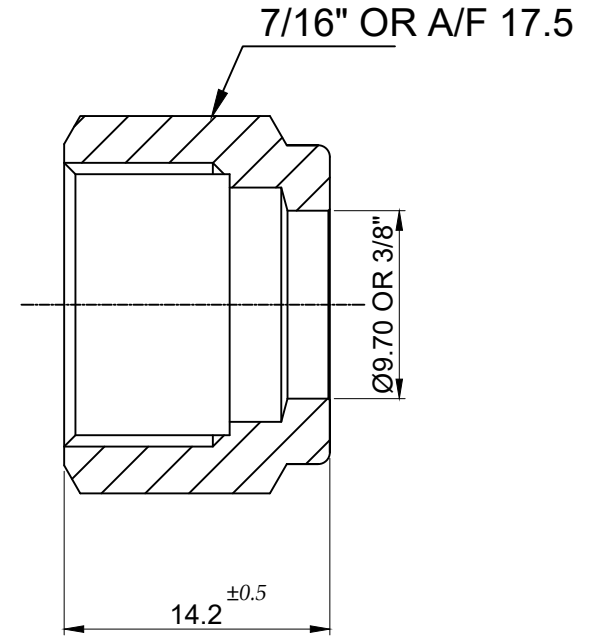
NUT
